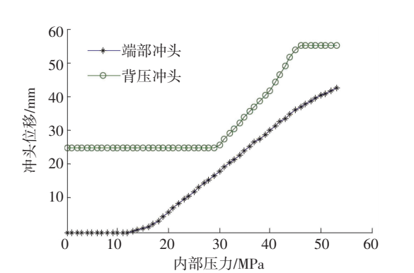
图 7 T 型 THF 仿真与试验加载曲线
