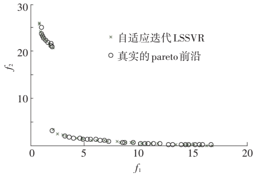
图 3 自适应迭代 LSSVR 模型与真实函数的 Pareto 前沿 Fig.3 The Pareto front obtained from adaptive iteration LSSVR and actual Pareto front
