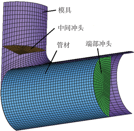
图 6 T 型 THF 有限元模型 Fig.6 A quarter of the finite element model used for numerical simulation
