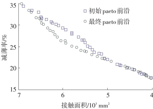
图 9 最终与初始 Pareto 前沿
