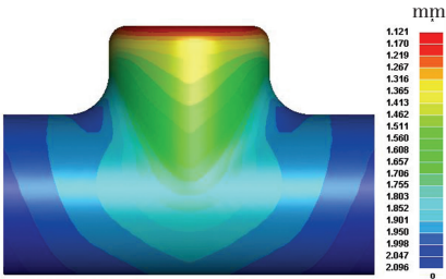
图 10 最优妥协解的厚度分布云图
