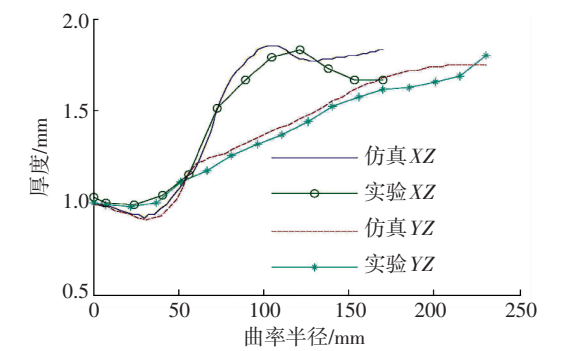
图 8 实验与仿真的厚度分布
